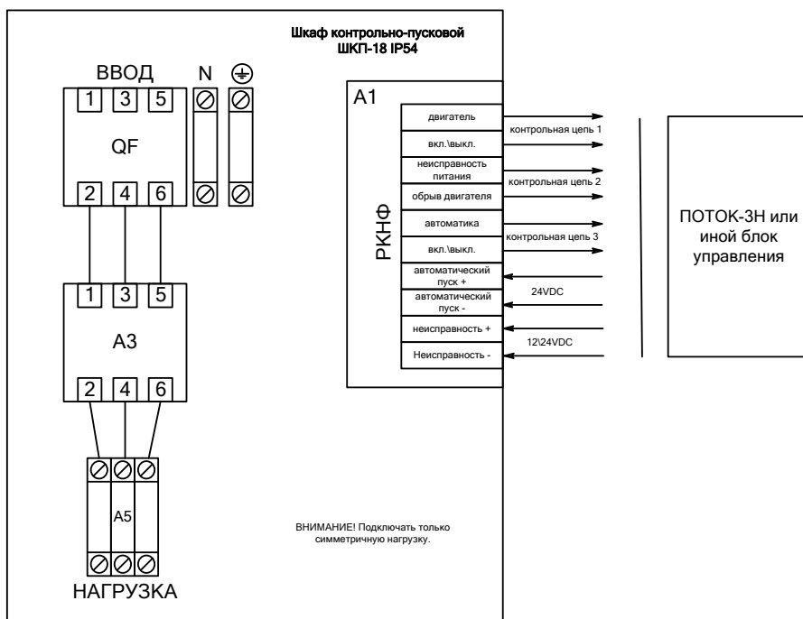
Рисунок 3. Схема электрическая подключения шкафа при эксплуатации
